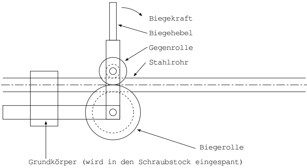
Rohr-Biegevorrichtung
