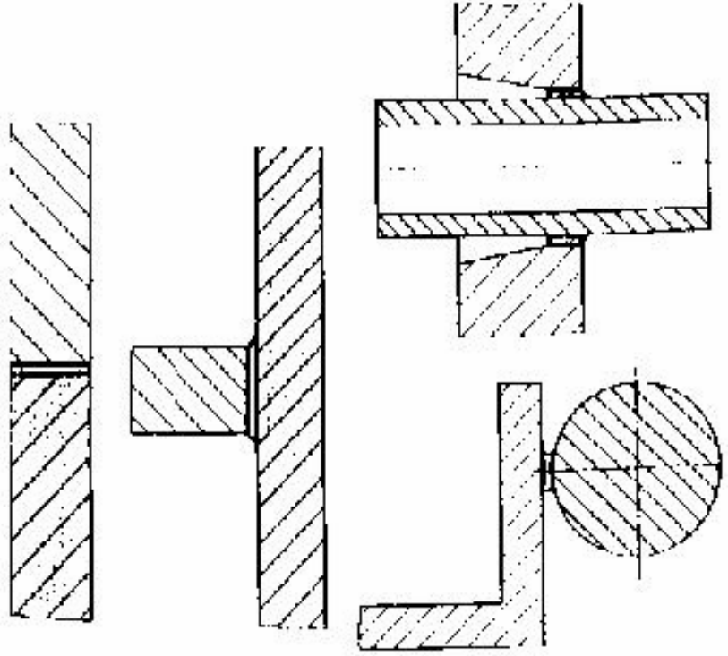
Schlechte Lötverbindungen:
