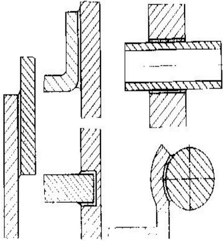
Gutgewählte Lötverbindungen:
